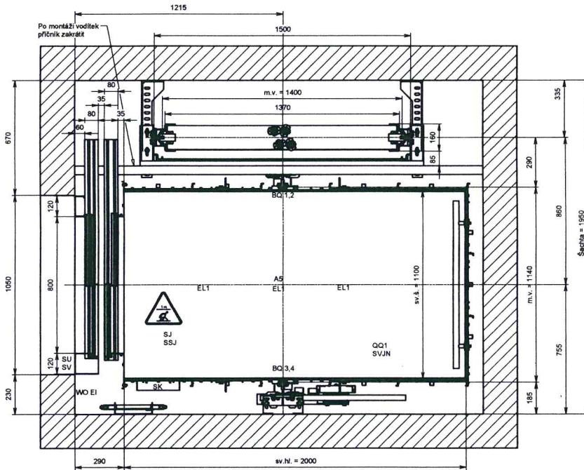
D-D (1:15)
