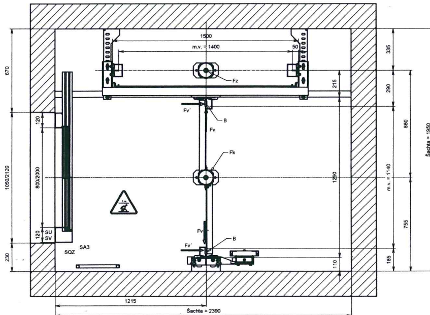
D-D (1:15)
