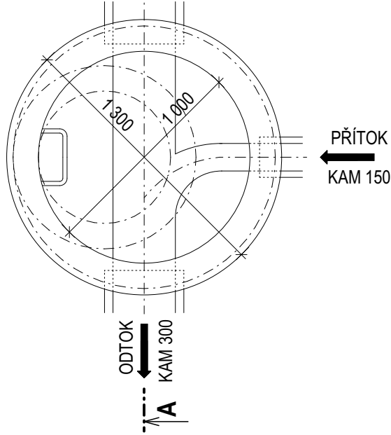
PŮDORYS:
