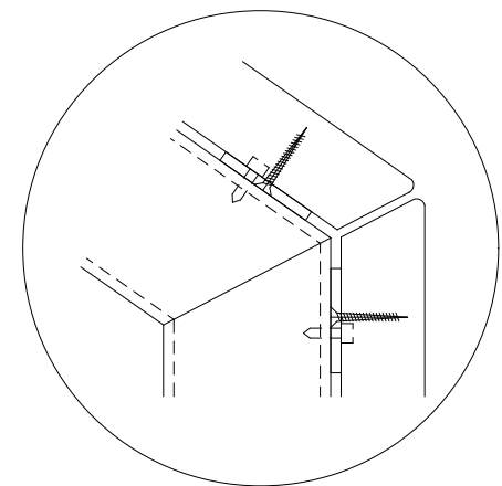
DETAIL SPOJE V NÁROŽÍ
